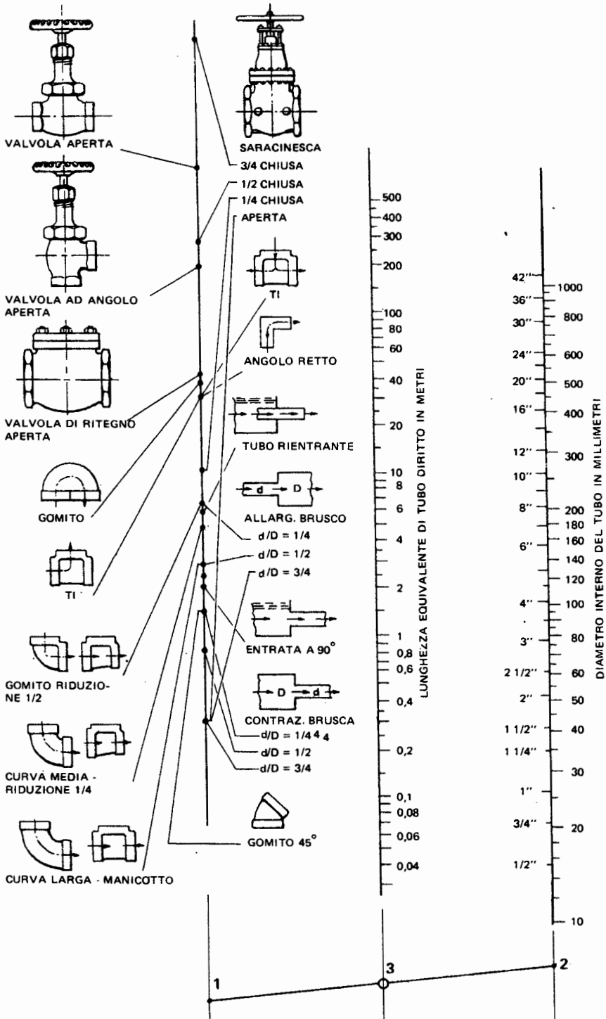
Fig. 35.24 - Abaco per la determinazione delle perdite di carico che si verificano al passaggio di acqua attraverso saracinesche, valvole, curve, variazioni di sezione, ecc.
